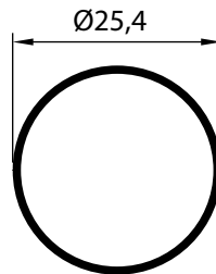
P-621 0,214 Kg/m
