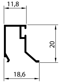
P-27 0,167 Kg/m
