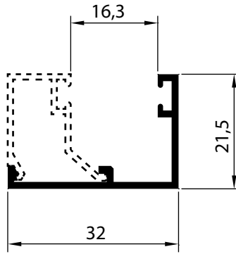
P-26 0,245 Kg/m
