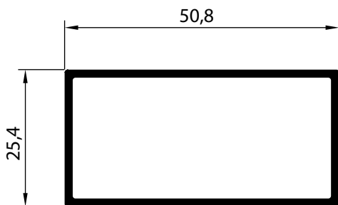
P-317 0,613 Kg/m
