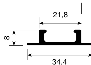
P-371 Perfil Inferior 0,227Kg/m 12 un/pacote
