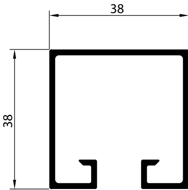
P-37 0,682 Kg/m
