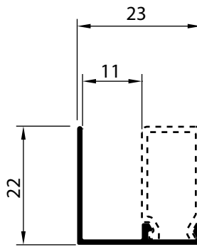
P-259 0,144 Kg/m
