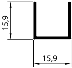
P-12 0,151 Kg/m
