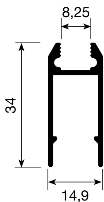
P-370 Perfil Leito 0,319 Kg/m 12 un/pacote
