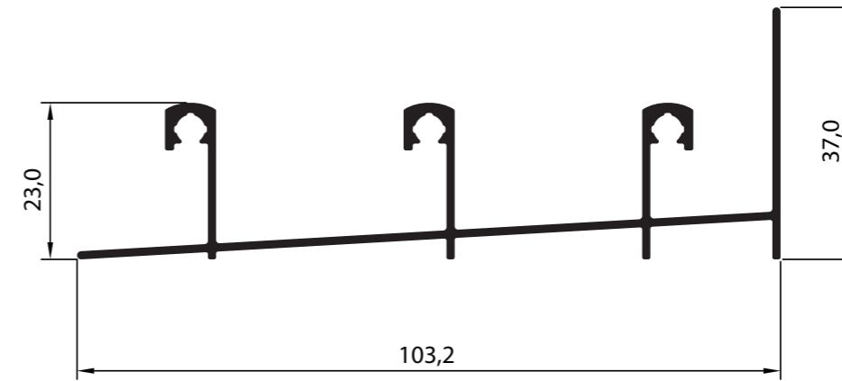
P-1281 Perfil SU 230 0,840 Kg/m
