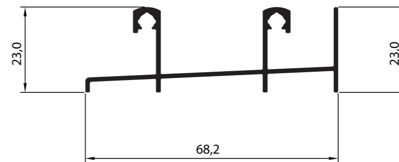
P-1286 Perfil SU 260 0,568 Kg/m
