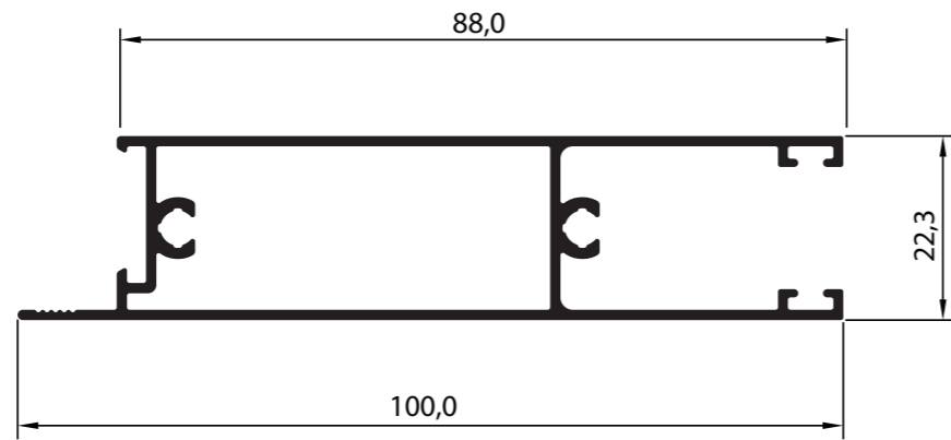
P-1278 Perfil SU 225 0,933 Kg/m
