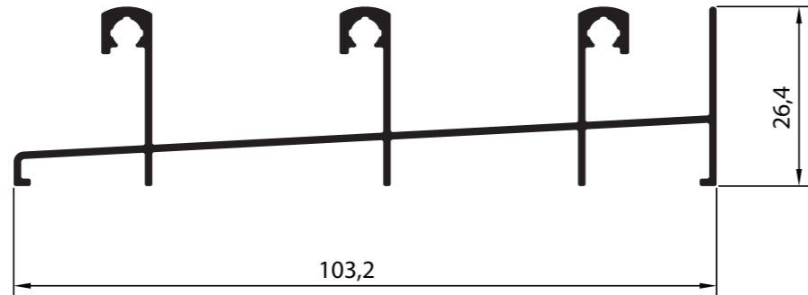
P-1260 Perfil SU 023 0,808 Kg/m
